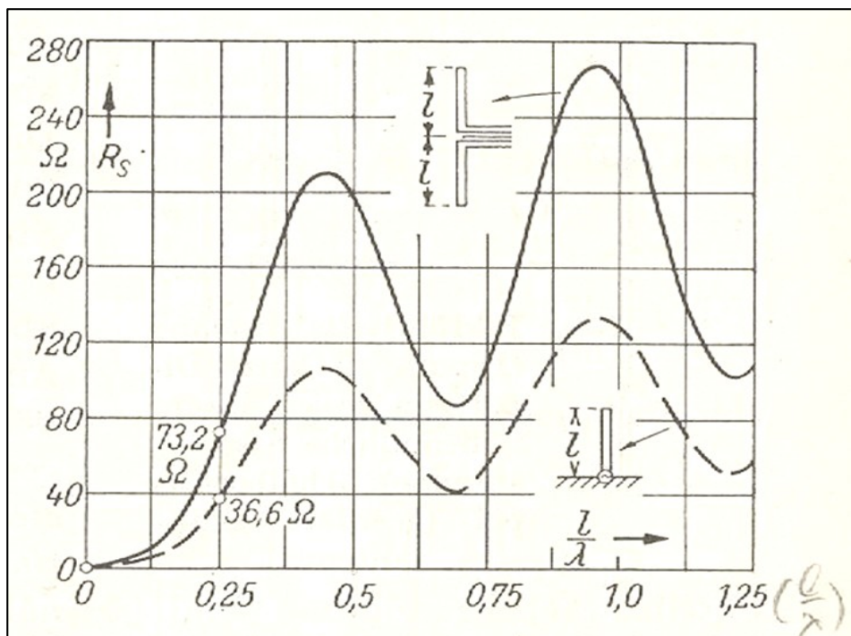
Bild 6: Strahlungswiderstand einer geraden Antenne bei verschiedenen Oberwellen aus Jahrbuch der Telegrafie. Van der Pol, Siegel und Labus, 13, 217, 1918. Für eine Antenne mit der Länge l = \lambda/2 beträgt der Strahlungswiderstand R_s = 73.2 \, \Omega . (Die Länge des Dipols ist hier als 2 \times l definiert!)
