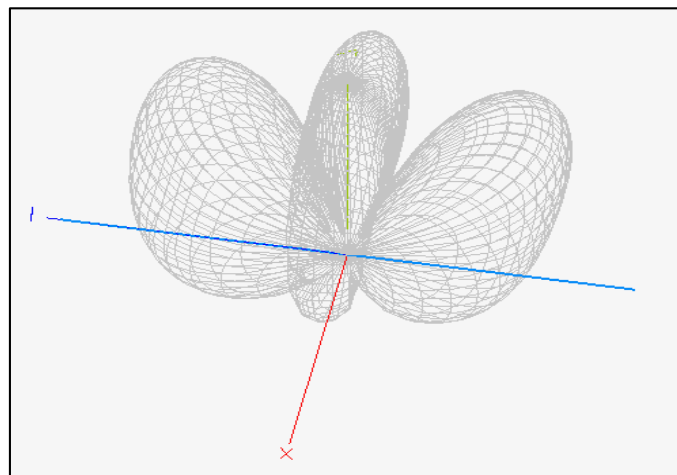
Bild 10 Räumliches Richtdiagramm der Horizontal-Antenne für k = 3 – siehe auch Bild 12 b.
