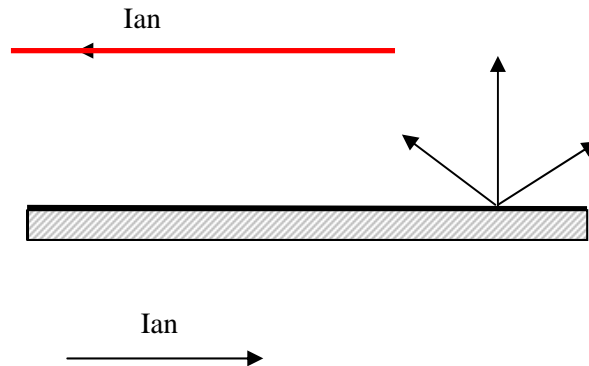
Bild 8: Strom in einer Horizontalantenne und Gegenstrom im Erdbereich (idealisiert).
