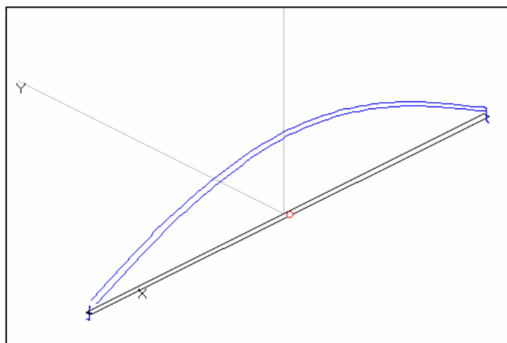
Bild 1: Stromverteilung auf dem Faltdipol bei Erregung in der Grundfrequenz f = 3.6 \text{ MHz}
