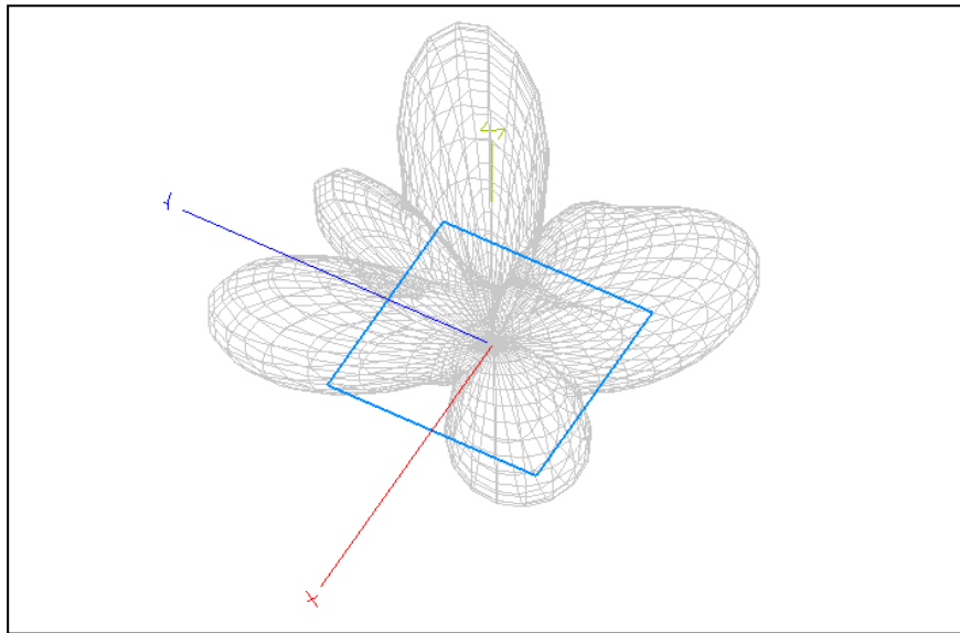
Bild 2: Fernfelddiagramm der liegenden Viereck -Schleife 4 x 21 m, f = 14.15 MHz
